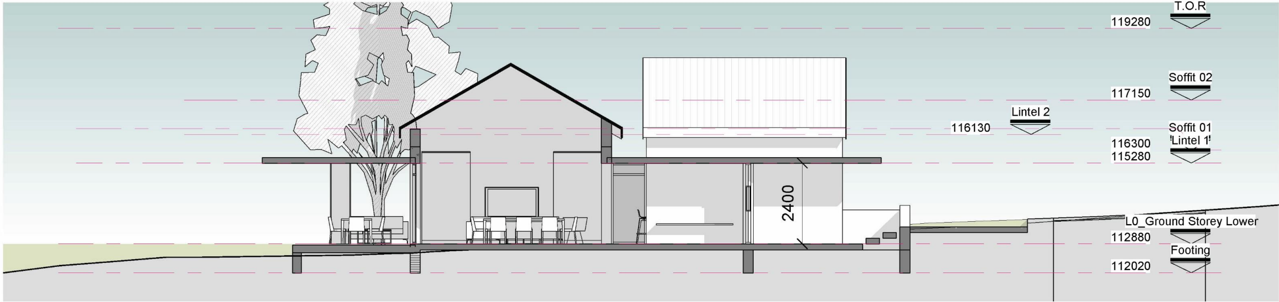
Section AA 1 : 100
