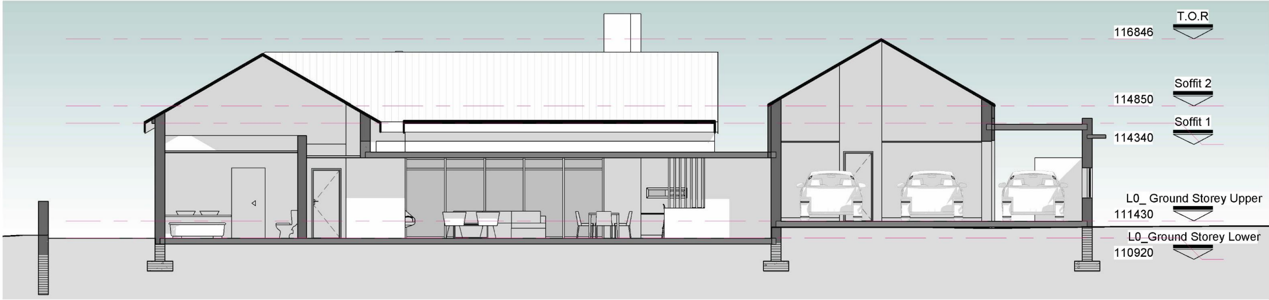
Section B-B 1 : 100
