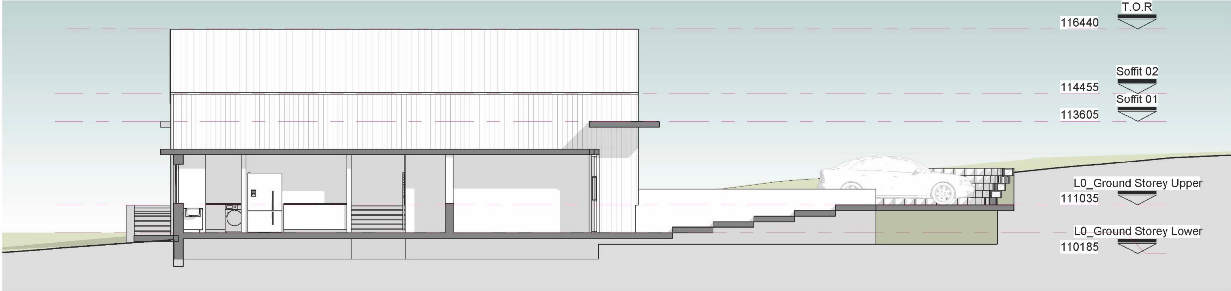
5-2 Section AA 1 : 100
